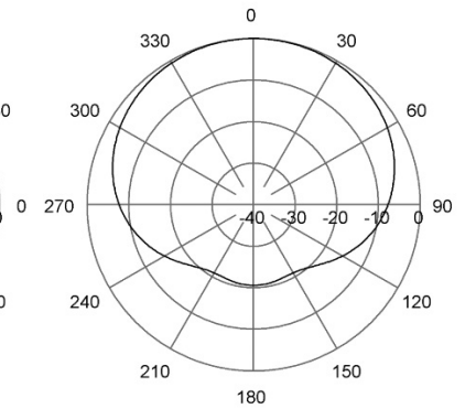
H-Plane | 71 MHz
