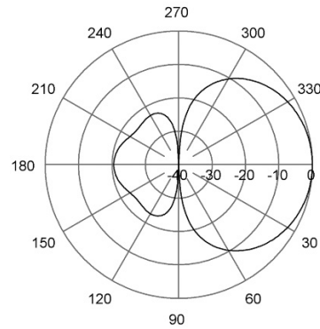
E-Plane | 71 MHz
